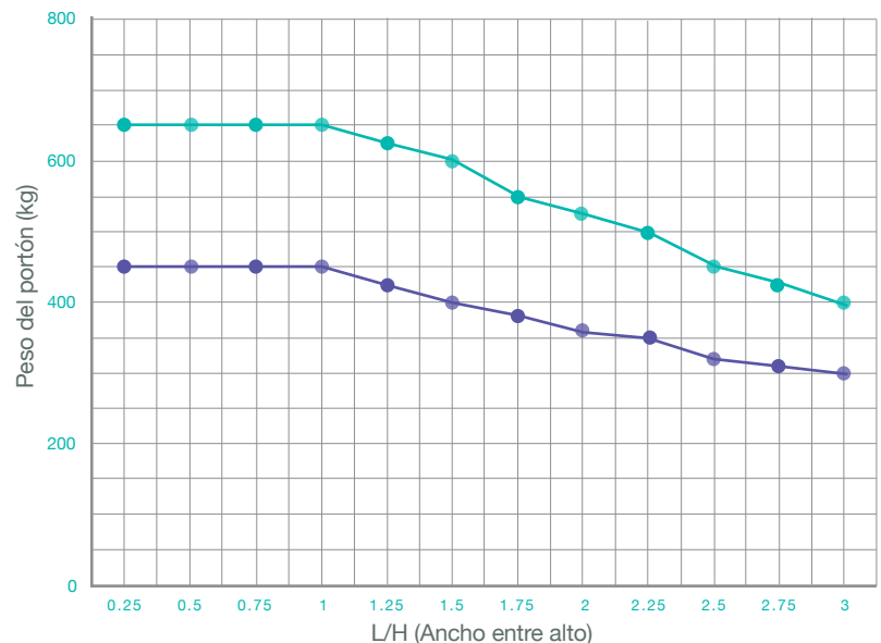
Límites de cargas según dimensiones (Bisagra Mediana Grande)
