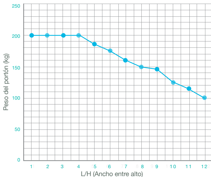
Límites de cargas según dimensiones (Bisagra Pequeña)
